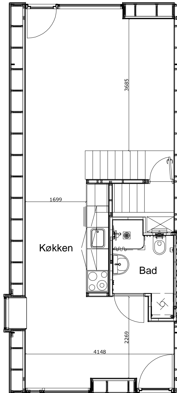
Stueplan
