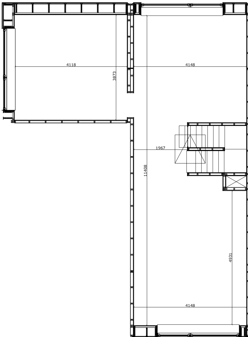
1. sal
