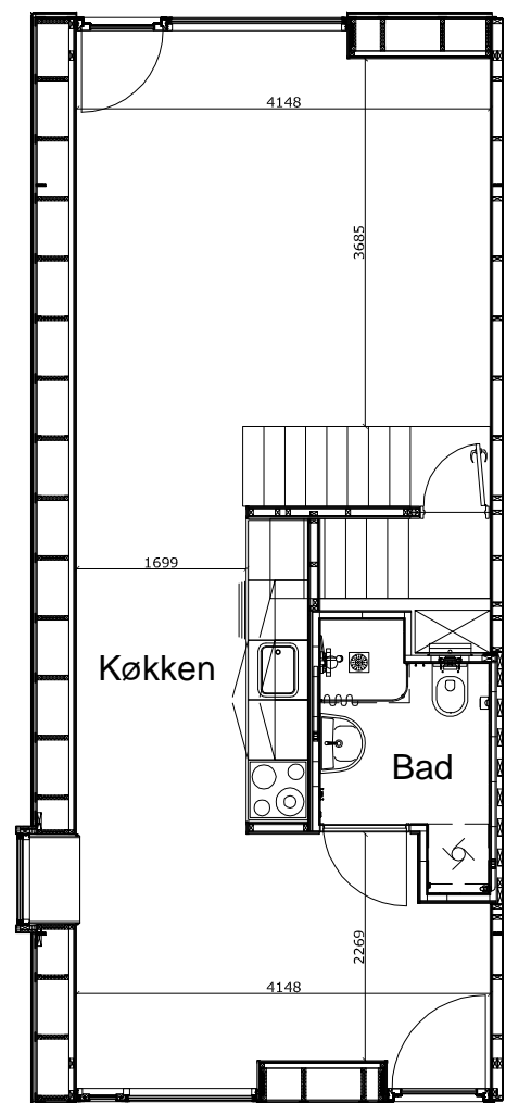
Stueplan
